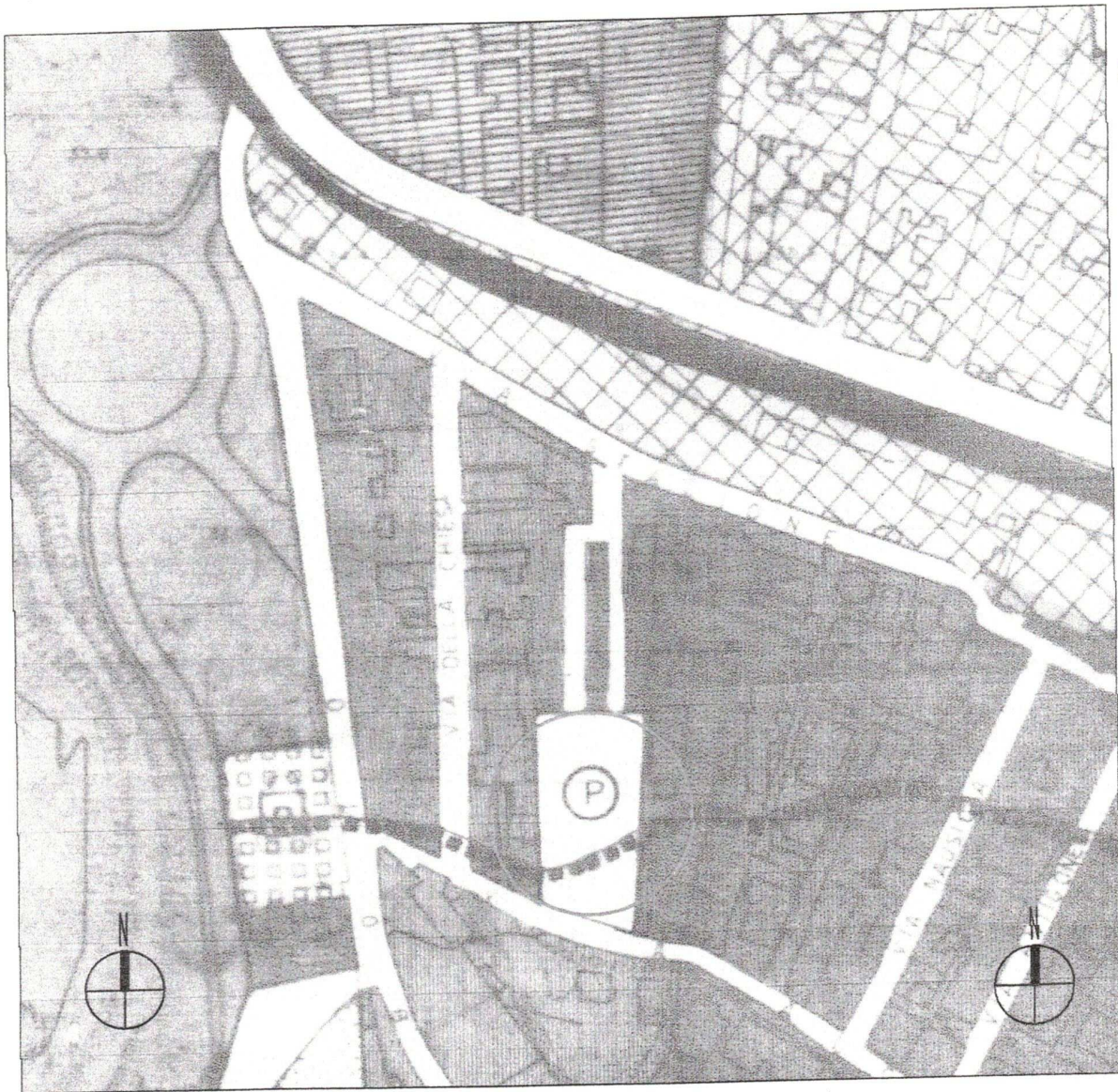
STRALCIO DEL PRG scala 1:2000
